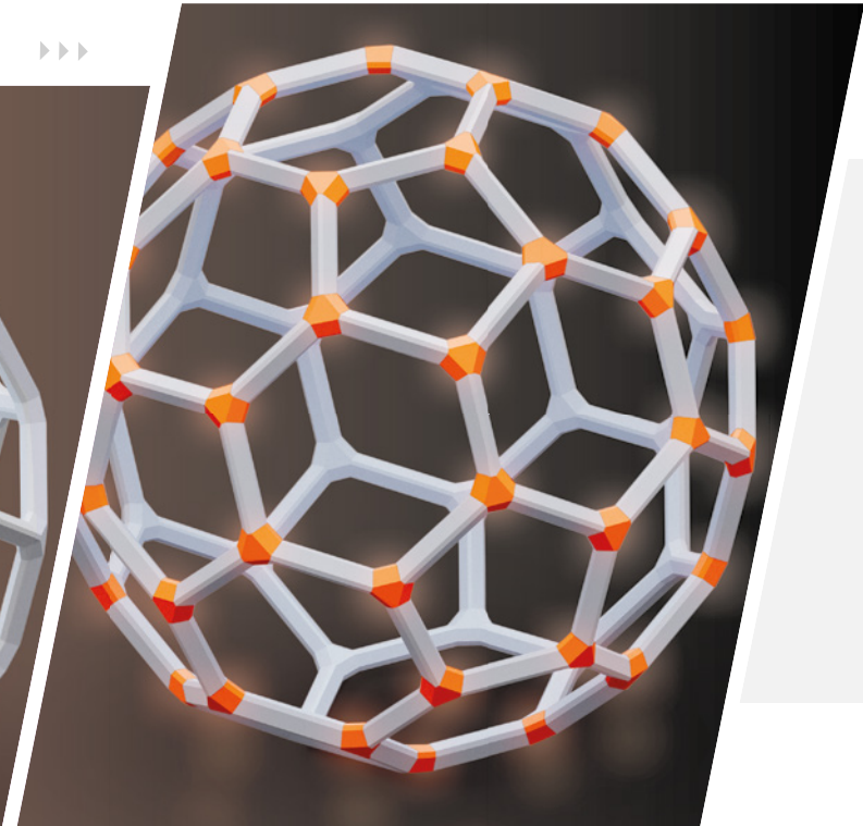
C 60 MOLEKÜL
